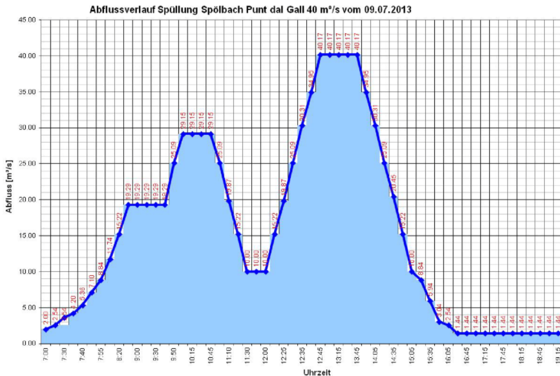
Abb. 6-1: Abflussverlauf der Spülung vom 09.07.2013 im Spöl mit der entsprechenden Anstiegs- und Abstiegskurven zwischen 07:00 und 19:15 Uhr (Aufzeichnung EKW).
