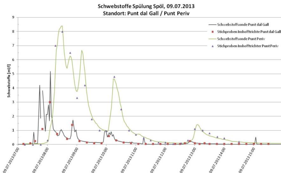
Abb. 6-2: Während der Spülung vom 09.07.2013 aufgezeichnete Schwebstoffmesswerte bei den Messstellen in Punt dal Gall und Punt Periv.
