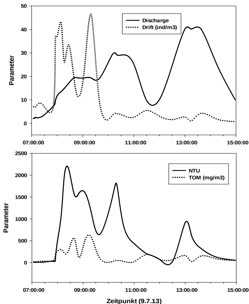
Abb. 6-3: Abfluss (Discharge, m^3/s ), Benthosdrift (Individuen/ m^3 ), Trübung (NTU) und transportiertes organisches Material (TOM: mg Trockenmasse/ m^3 ) während der Regenerations-Spülung am 9. Juli 2013.
